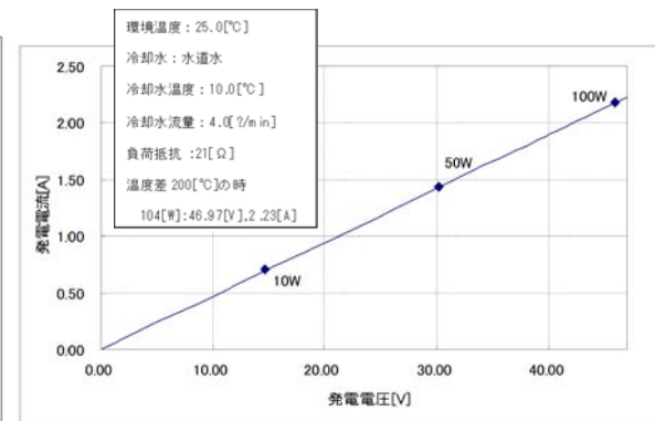
発電量に対する電圧値及び電流値
