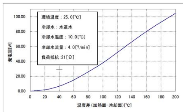
温度差に対する発電量
